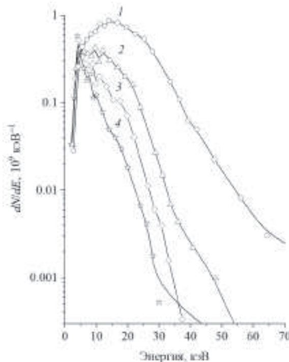
Рис. 12. Энергетический спектр ионов железа: 1 (○) — \text{Fe}^{14+} , 2 (Δ) — \text{Fe}^{12+} , 3 (◇) — \text{Fe}^{11+} , 4 (☆) — \text{Fe}^{10+} .
