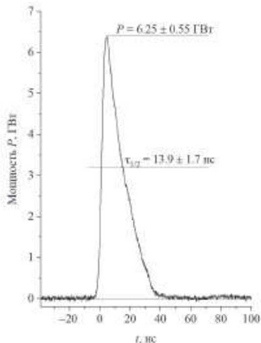
Рис. 5. Типичная форма импульса на выходе системы ФОКУС.
