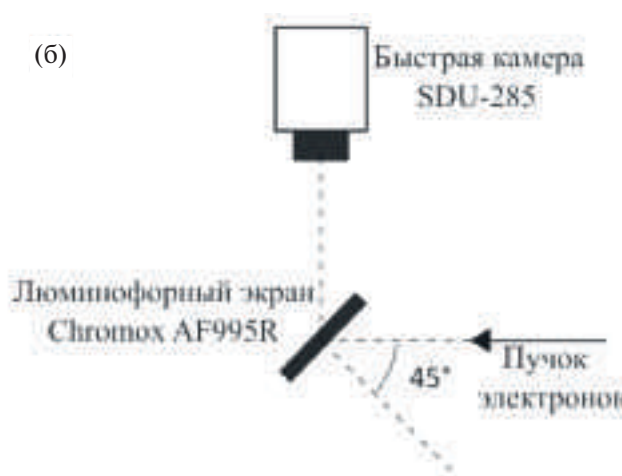
Рис. 6. а — Внешний вид флуоресцентного экрана Chromox с напылением золота толщиной 300 нм. б — Схема регистрации распределения тока пучка по излучению прошедшему сквозь пластину сцинтиллятора.
