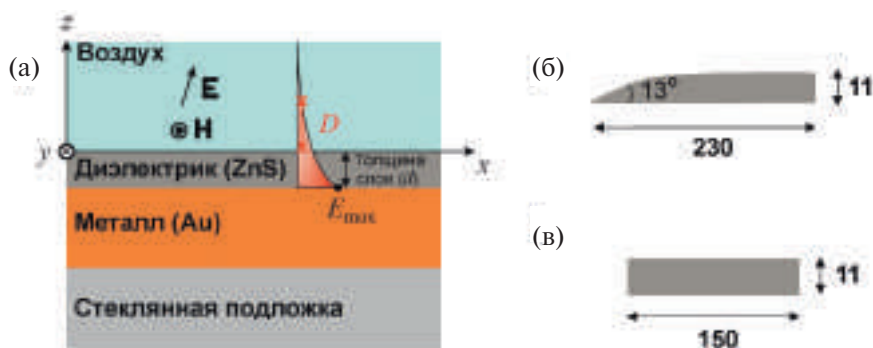
Рис. 4. а – Схемы структур образцов: x – расстояние от входного торца образца, z – расстояние от зонда до поверхности образца, D – глубина проникновения поля ППП в воздух, d – толщина покровного слоя ZnS, E и H – напряженности электрического и магнитного полей ППП соответственно; б и в – геометрия профилей образцов, используемых в зондовом методе и методе экранирования соответственно.
